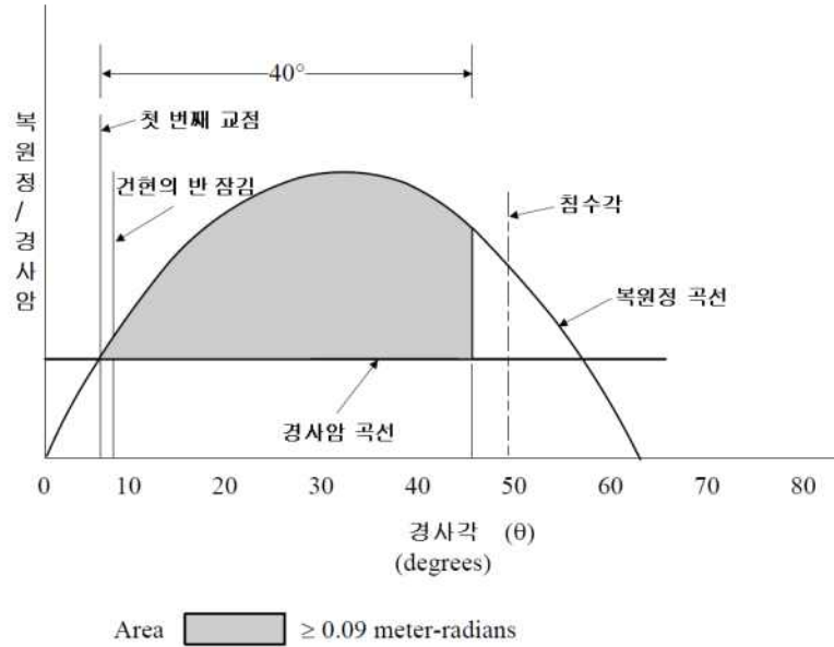
그림 8.2 복원정 및 경사압 곡선
