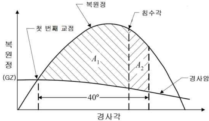
그림 5.1 복원정 및 경사암 곡선
